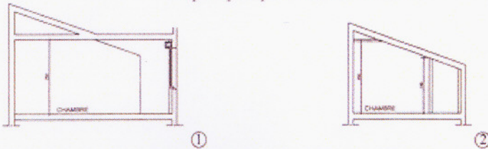
Coupe de principe sur chambre sous-toiture
